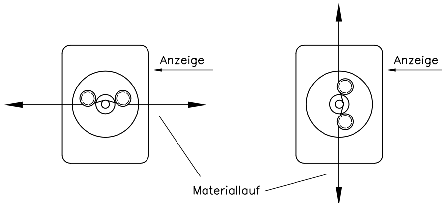
Ansicht A
